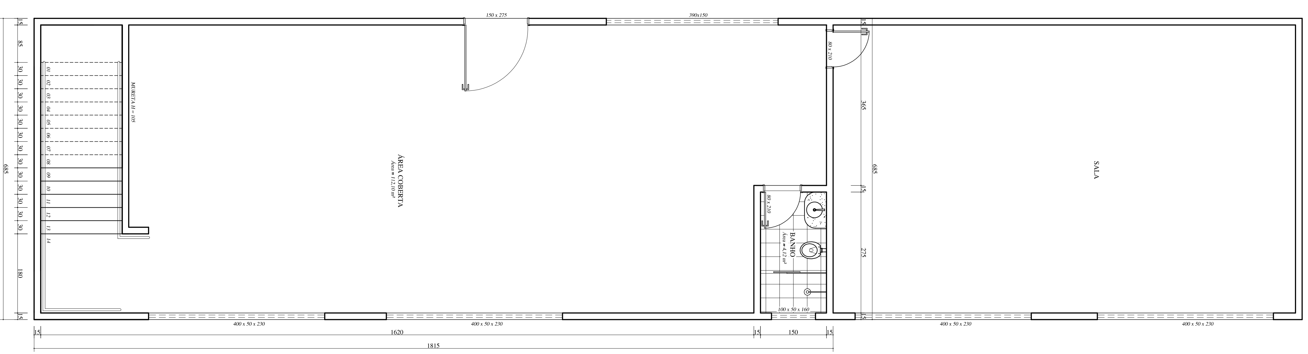
Planta Baixa - 1º Pavio Esc. 1:50 Área = 124,39 m 2
